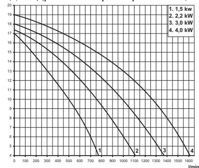
Н(м) Гидравлич. характеристики 1,5-4,0 кВт
